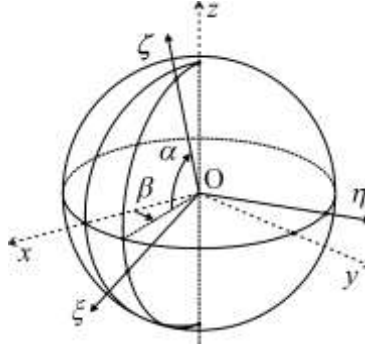
図2 絶対座標系と共通の原点を持つ一般の回転運動座標系
