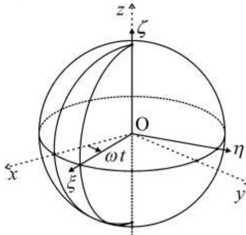
図3 絶対座標系 (O-xyz 座標系) と運動座標系 (O- \xi\eta\zeta 座標系)
