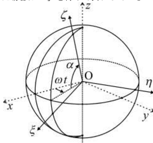
図 4 絶対座標系 (O-xyz 座標系) と運動座標系 (O- \xi\eta\zeta 座標系)
