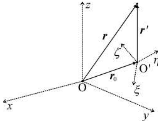
図 7 絶対座標系（O-xyz 座標系）と異なる原点を持つ運動座標系（O'-ξηζ 座標系）
