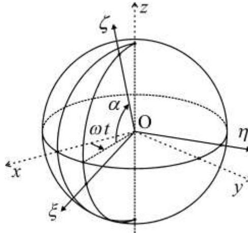
図 5 絶対座標系 (O-xyz 座標系) と運動座標系 (O-ξηζ 座標系)
